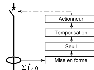
Fig. 24 : schéma fonctionnel d'un DDR.
