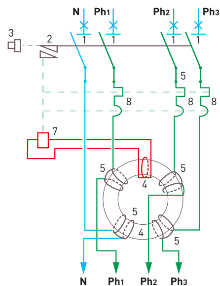
Disjoncteur tétrapolaire
