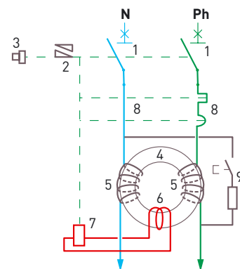
Disjoncteur Uni + Neutre
