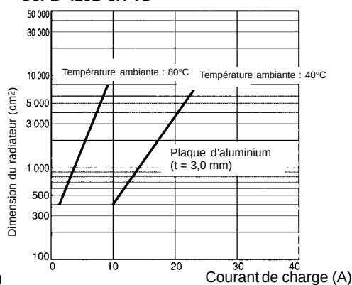
G3PB-425B-3H-VD
